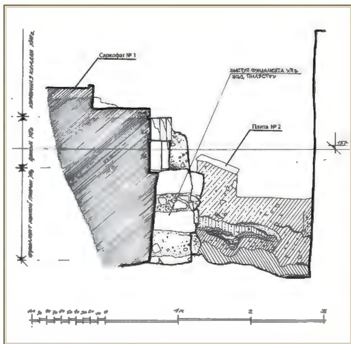
Рис. 8. Южная галерея: разрез участка кладки с дном саркофага № 1 (по оси север-юг, вид с востока)
